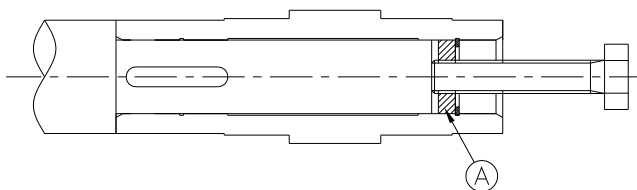
A部断面図
